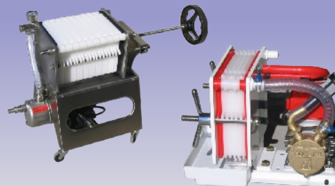
Lapszűrők, 20x20 cm-es lapokkal, szivattyúval szerelve. Rozsdamentes vagy festett kivitelben 250 l/óra teljesítménytől.
